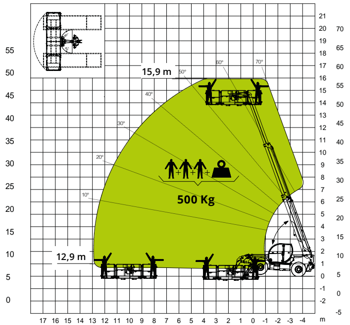
Diagramma portate cestello estensibile 500 kg
