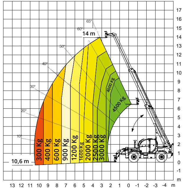
Diagramma portate su pneumatici
