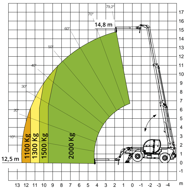
Diagramma portate Jib 2.000 kg
