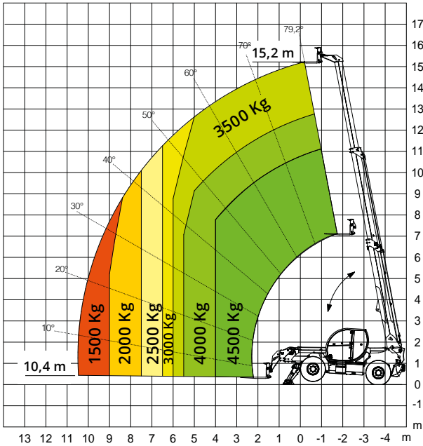
Diagramma portate su stabilizzatori
